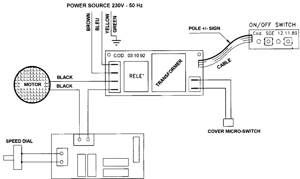
ABB.Nr.6 - Einphasiges elektrisches Schema ZERKLEINERER mit Regler
